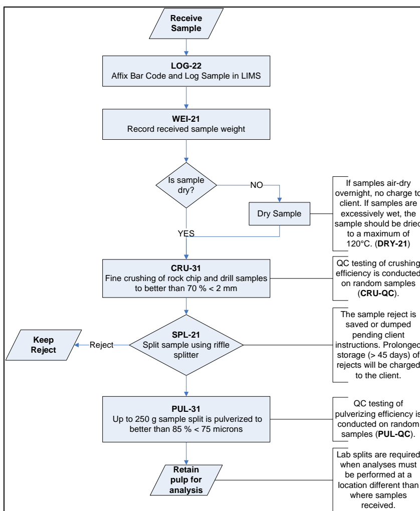
Figure 13.1 ALS Chemex - Sample Preparation Procedure
